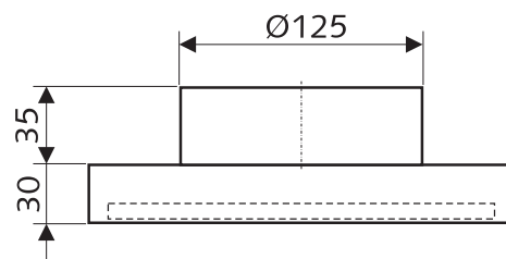
Ansicht Drosselelement
